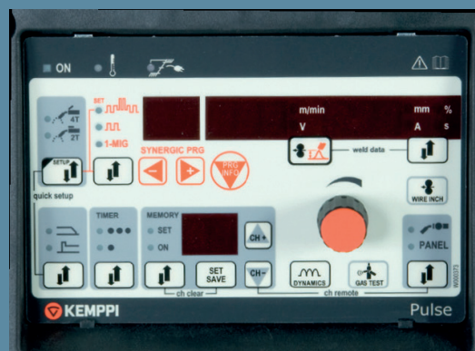
Kempact Pulse 3000 - ovládací panel.
